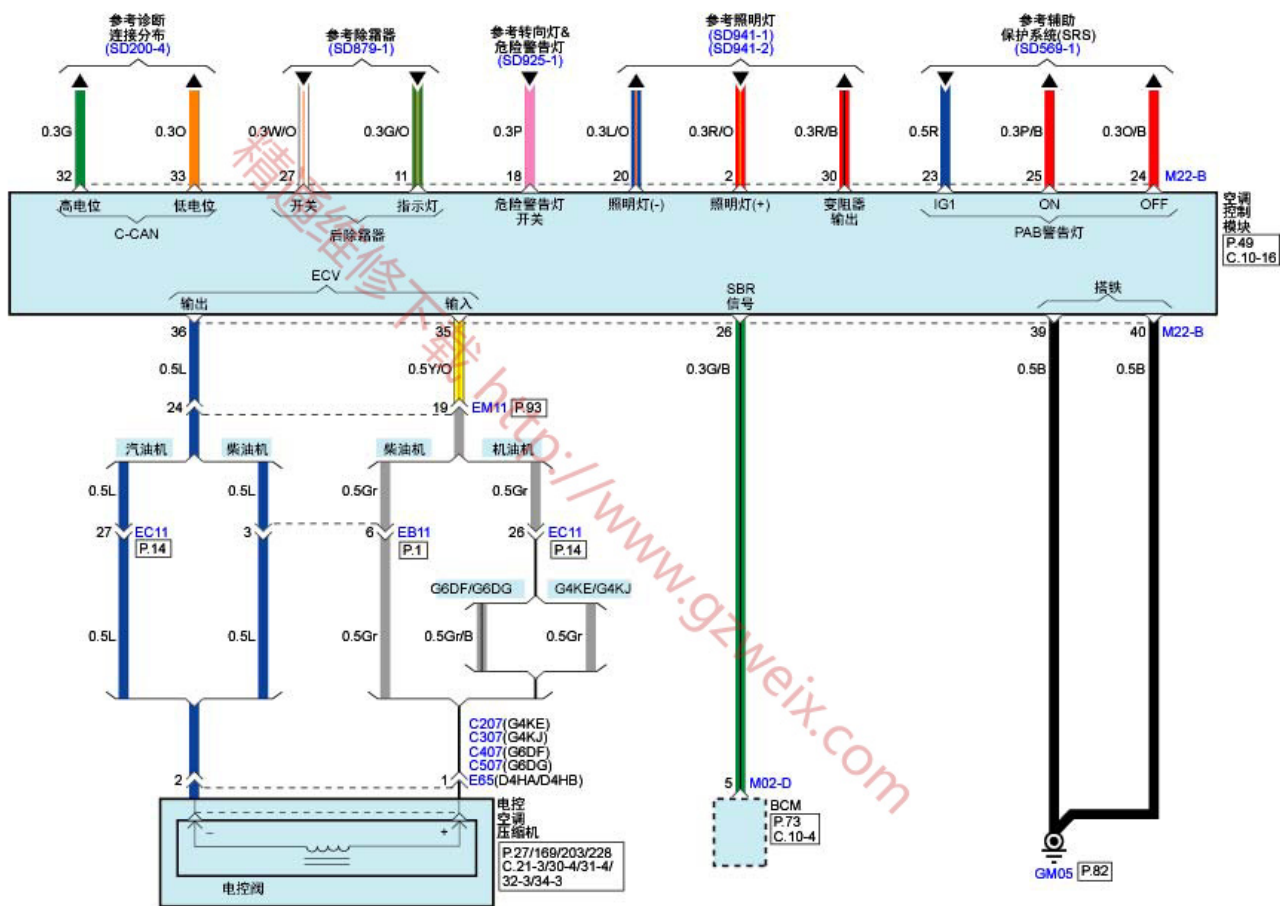
空调控制系统(手动)(3)
